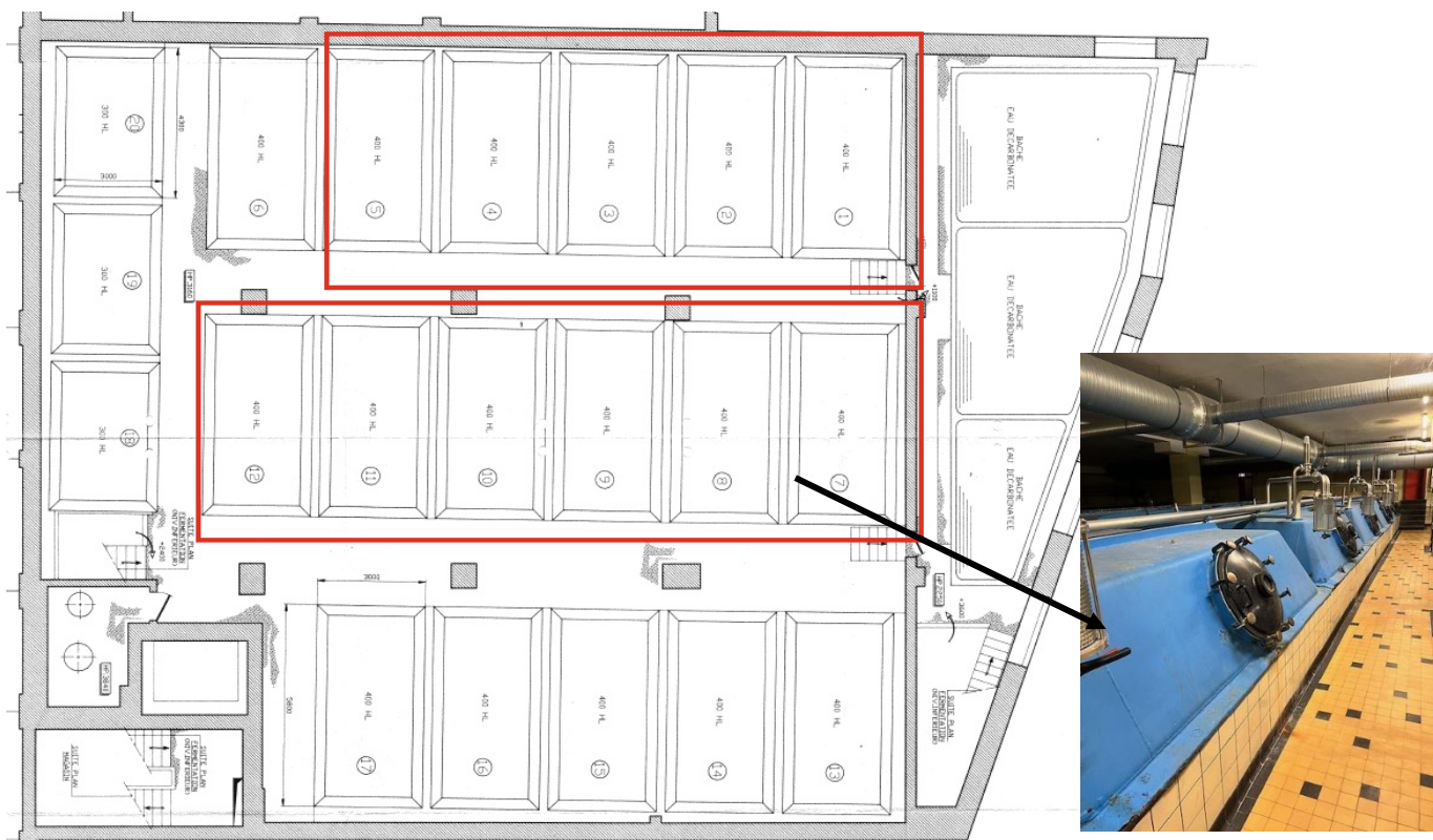
Figure 6 : Localisation des anciennes cuves – atelier siroperie
